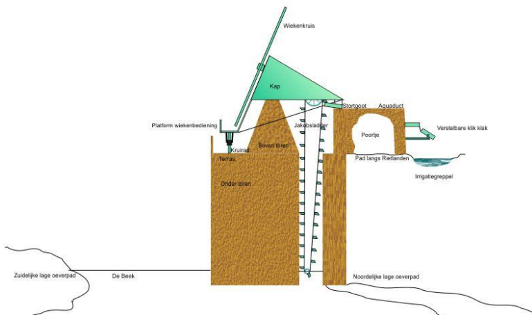
Wind irrigatiemolen doorsnede – elektronische tekening Micha Beuger
